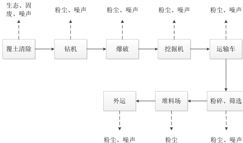
图1.1 原项目生产工艺流程图
